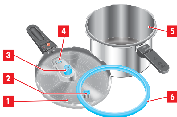
Fig. 3: Parte inferiore del coperchio in dettaglio
