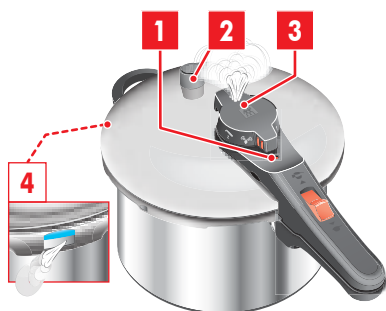
Fig. 1: Funzioni di sicurezza
