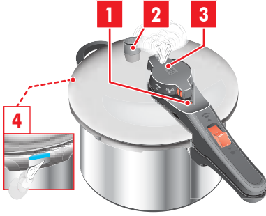
Resim 1: Emniyet fonksiyonları
