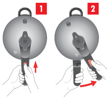
Рис. 5: Снятие крышки
