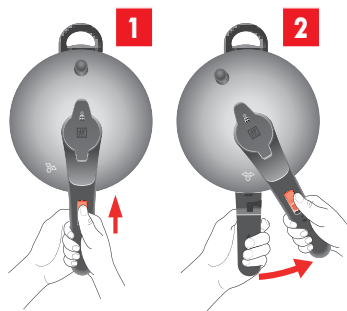
Abb. 18: Deksel openen
