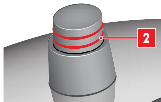
Abb. 14: Garstufe kontrollieren
