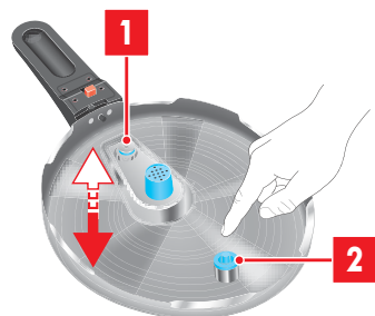
Fig. 10: Comprobaciones de seguridad
