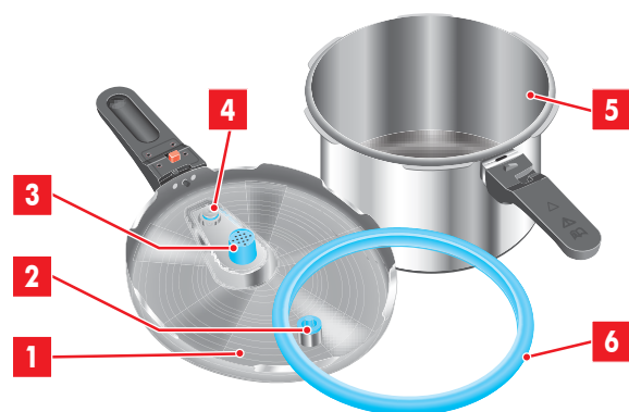
示意图 3: 锅盖底面细节图
