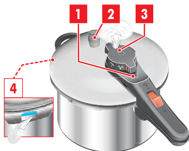
Fig. 1: Sikkerhedsfunktioner
