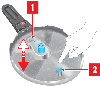
그림 8: 안전 점검
