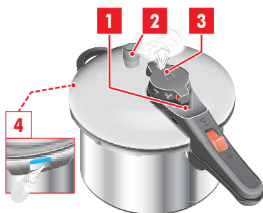
Abb. 1: Veiligheidsfuncties
