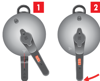
그림 10: 뚜껑 닫기
