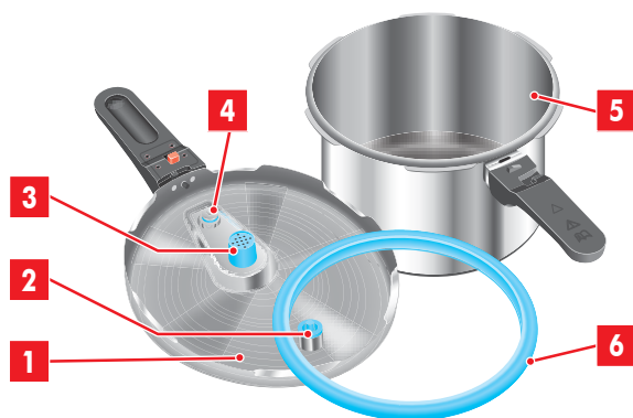
Fig. 3: Detaljeret fremstilling af lågets underside
