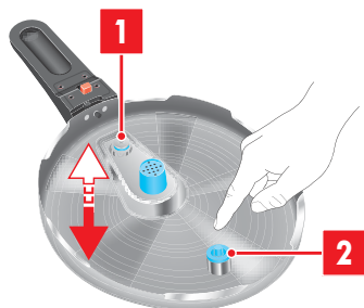
Рис. 11: Проверки функций безопасности
